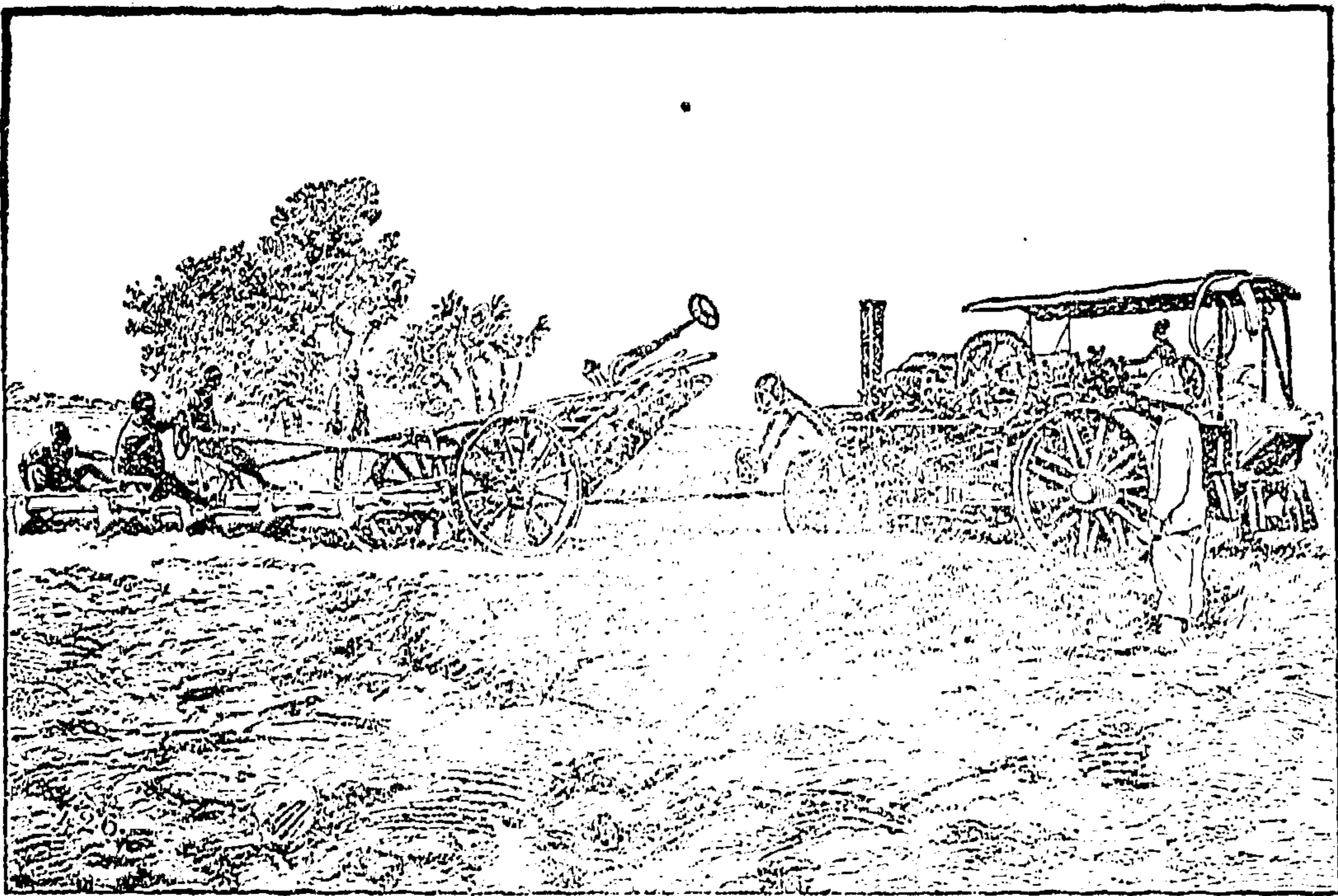
Kemnas Heißdampfplüg auf einer Plantage in Kingwangwanda der Deutschen Rufiji Baumwoll-Gesellschaft in Tätigkeit.
