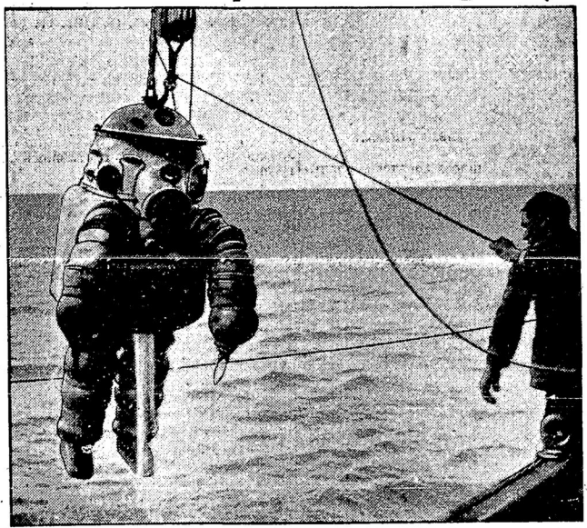
Въ Адриатическомъ морѣ у восточныхъ береговъ Италіи водолазы извлекаютъ цѣнные грузы съ кораблей, пущенныхъ ко дну во время великой войны германскими и австрийскими подводными лодками. — Водолазы въ особомъ аппаратѣ, предназначенномъ для большихъ глубинъ, опускаются на дно.
