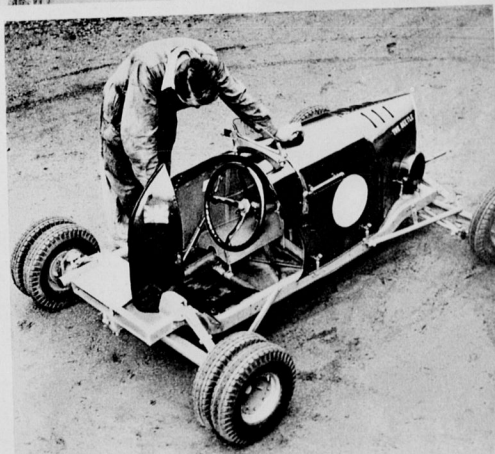
Ein von dem Engländer H. D. Killick konstruierter Rennwagen, der sich für Bergrennen besonders eignen soll und für das gestrige „Shelsby Walsh“ bestimmt war. Die Anfangsgeschwindigkeit soll verhältnismässig gross sein, der Stundendurchschnitt jedoch nur bis zu 130km. Die Ausmasse des Wagens scheinen erstaunlich klein!
