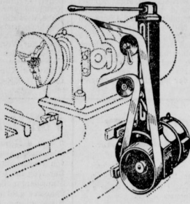
A.E.G.-Flanschmotor-Stufengetriebe
